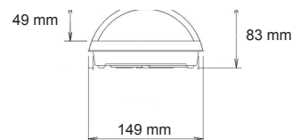
UniLED enkelsidig
