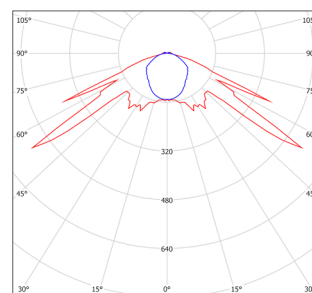
UniLED dubbelsidig
